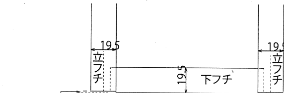
縁下部詳細図(正面から見た図)
