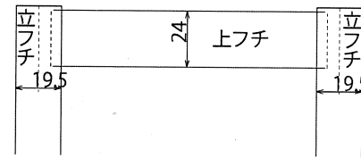
縁上部詳細図(正面から見た図)
